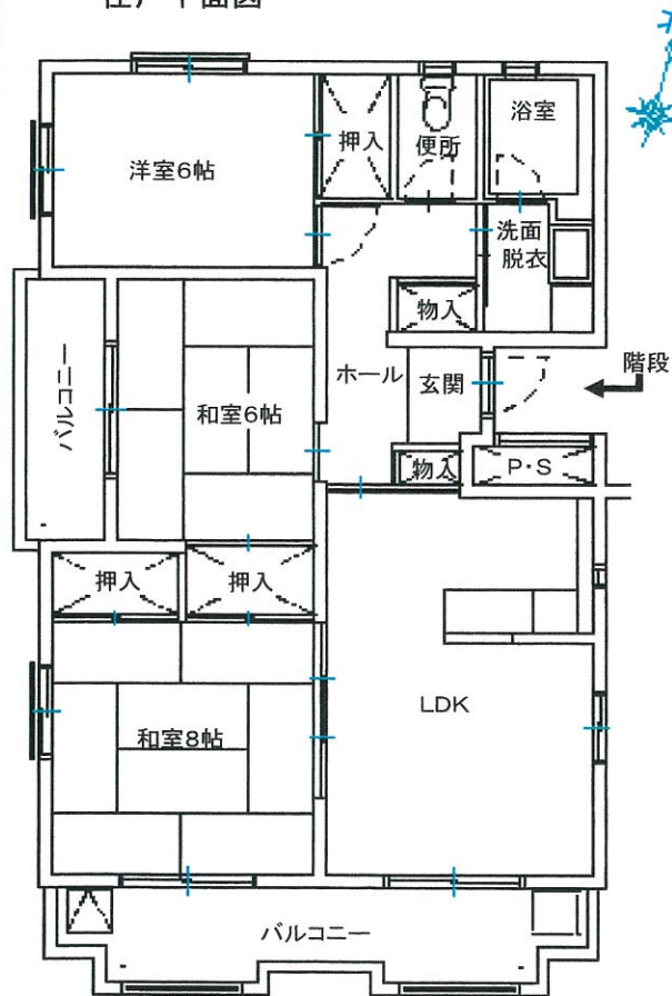
住戸平面図
