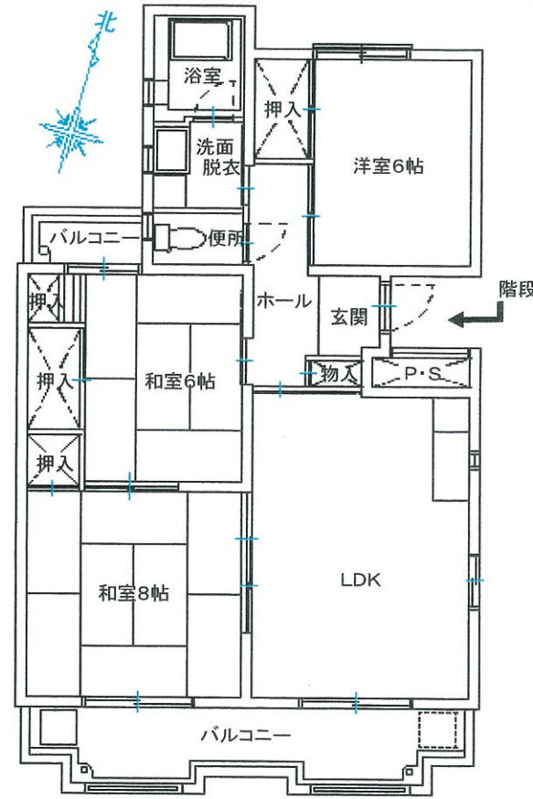
住戸平面図(部屋番号末尾奇数は反転)
