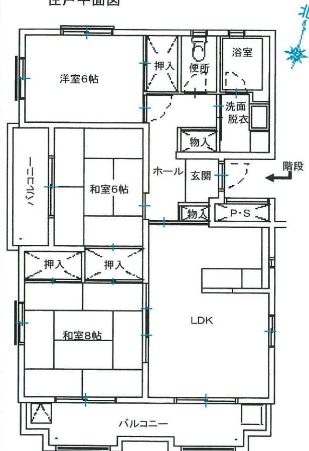
住戸平面図
