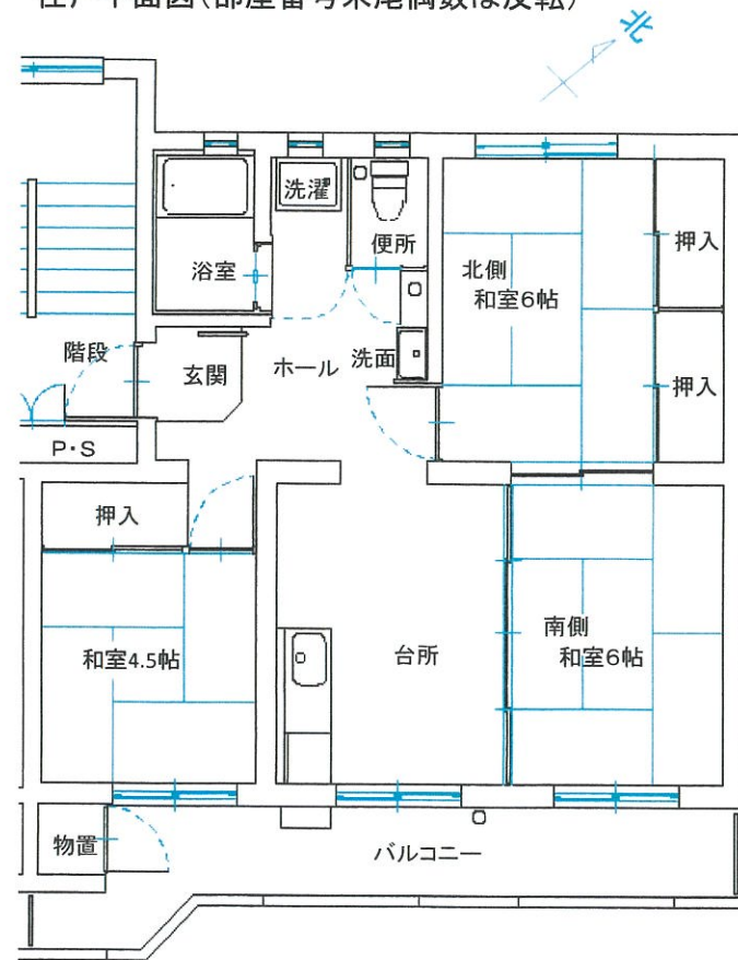
住戸平面図(部屋番号末尾偶数は反転)
