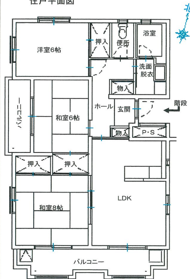
住戸平面図
