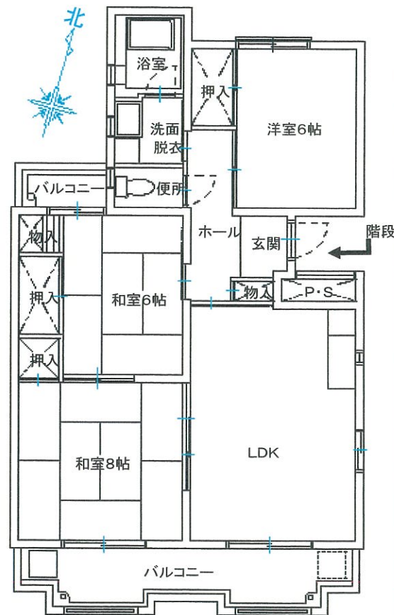
住戸平面図(部屋番号末尾奇数は反転)
